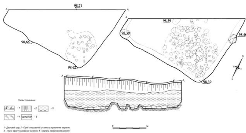
Рис. 7. Загірці V. План та стратиграфічний перетин об'єкта 6.
