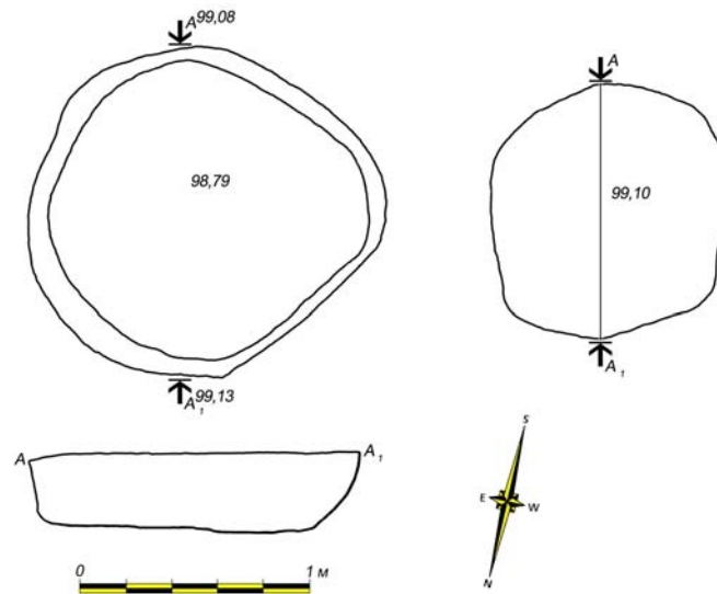
Рис. 1. Загірці I. План об'єкта 3 на рівні виявлення та після вибирання заповнення.
