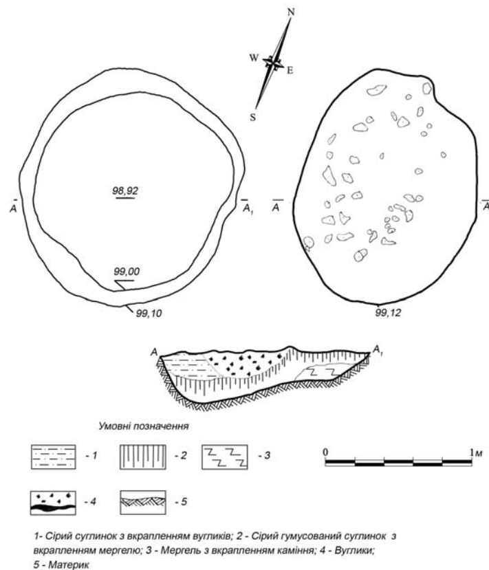
Рис. 6. Загірці V. План та стратиграфічний перетин об'єкта 4. Fig. 6. Zahirtsy V. Plan and stratigraphy profile of object 4.
