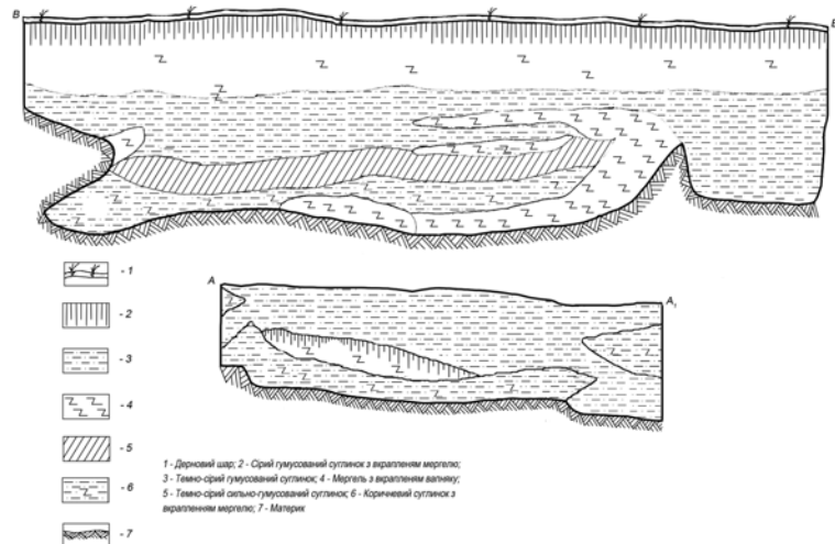
Рис. 5. Загірці V. Стратиграфічний перетин об'єкта 3. Fig. 5. Zahirtsy V. Stratygraphy profile of object 3.
