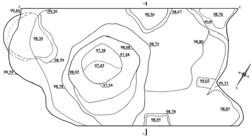
Рис. 4. Загірці V. План об'єкта 3 після вибирання заповнення. Fig. 4. Zahirtsy V. Plan of object 3 after excavations.
