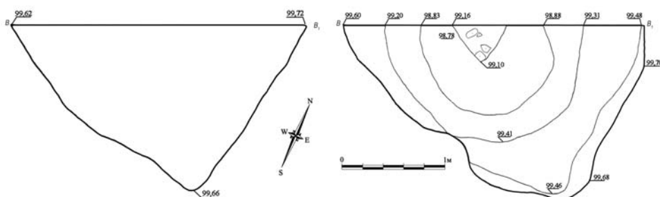
Рис. 2. Загірці V. План об'єкта 2 на рівні виявлення та після вибирання заповнення. Fig. 2. Zahirtsy V. Plan of object 2 on the detection level and after excavations.
