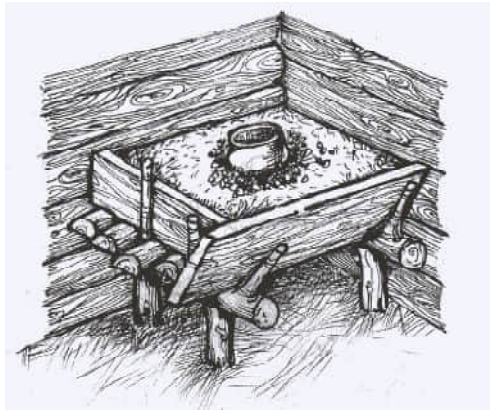
1. Відкрите вогнище (“горно”) у с. Можари Овруцького р-ну Житомирської обл. (реконструкція автора за матеріалами М. Брицуна-Ходака)
